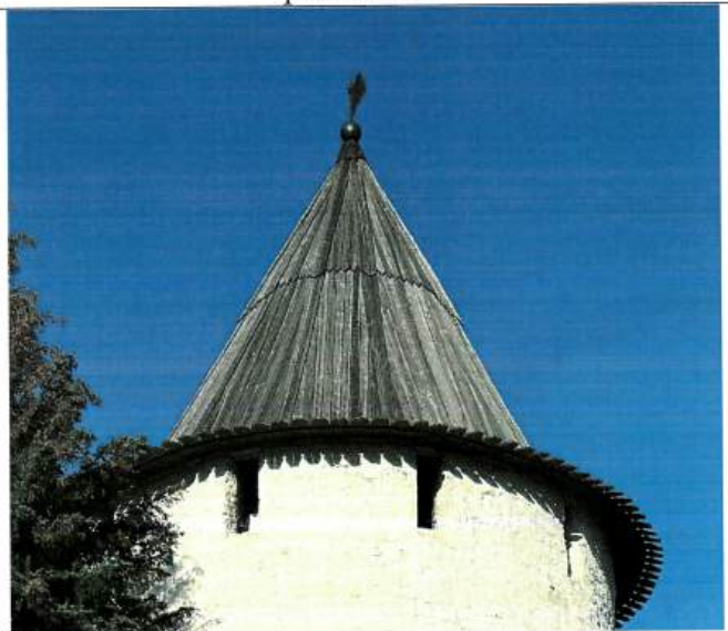
Рис. 14. Шатровая тесовая кровля с полицами, металлический прапор.
