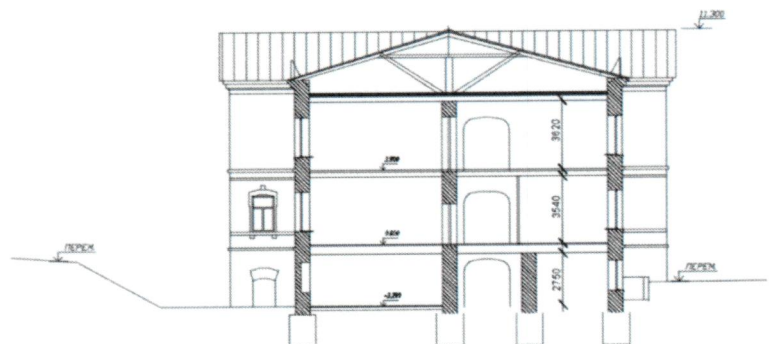
Разрез
