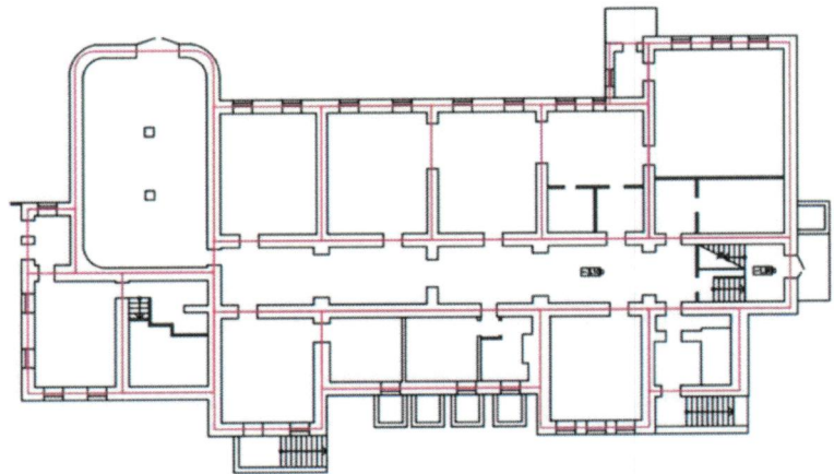
План подвала
