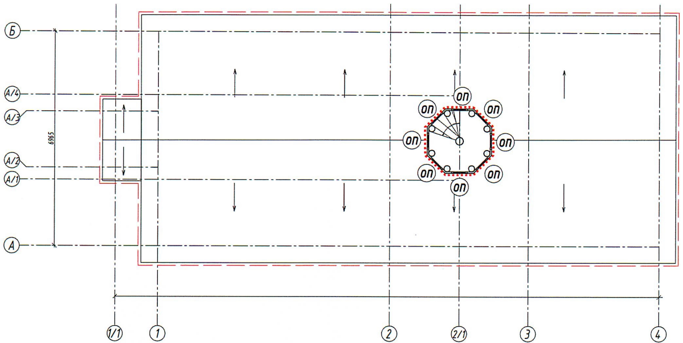
План чердака
