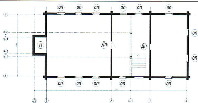
План 1 этажа (Графическая схема №2)
