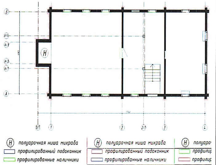
План 1 этажа (Графическая схема №2)
