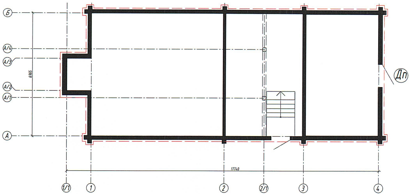
План подклета
