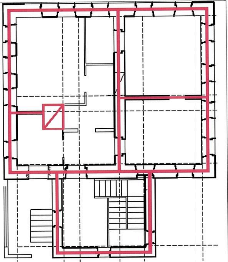
План 1 этажа.
