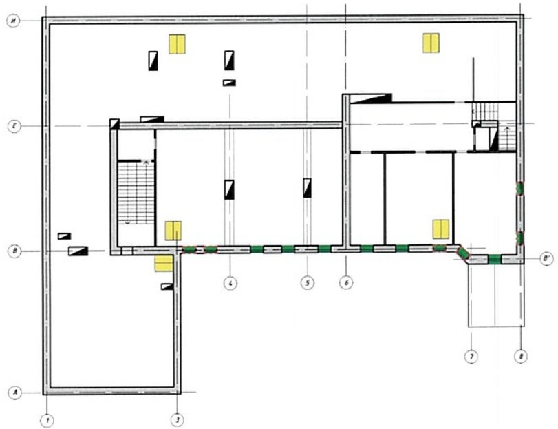
Схема расположения исторических проемов и столярных заполнений антресольного этажа с чердаком.
