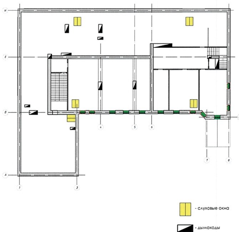
План чердака с обозначением исторических мест расположения слуховых окон и дымоходов
