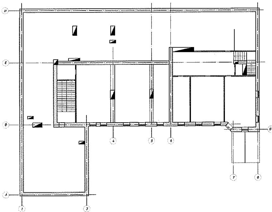
План чердака и антресольного этажа
