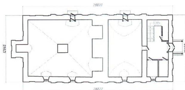
Месторасположение, пропорции и геометрия оконных и дверных проемов
