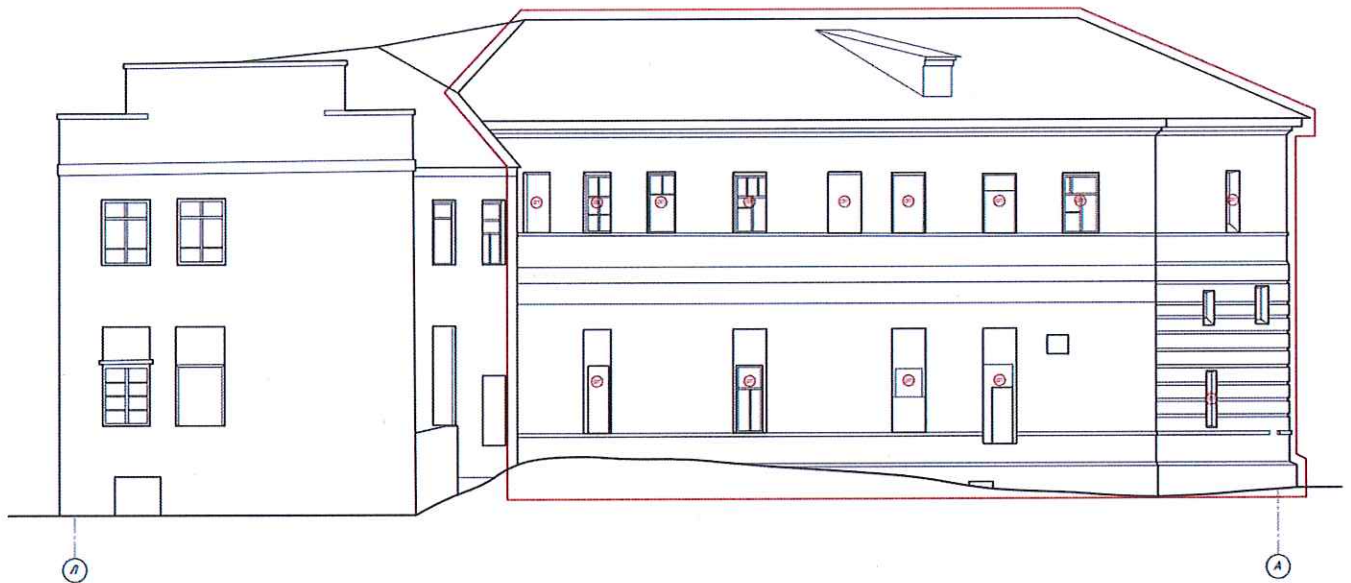
Графическая схема №5. Фасад в осях Л-А.
