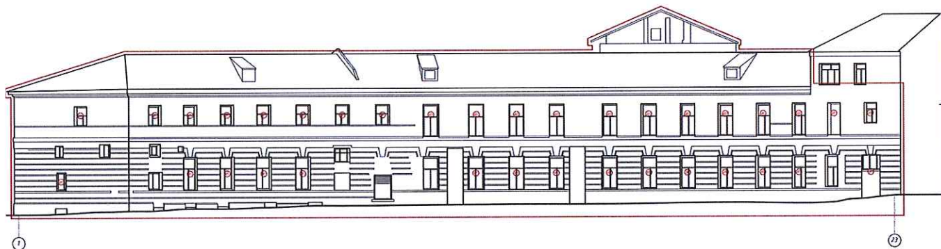
Графическая схема №4. Фасад в осях 1-23.
