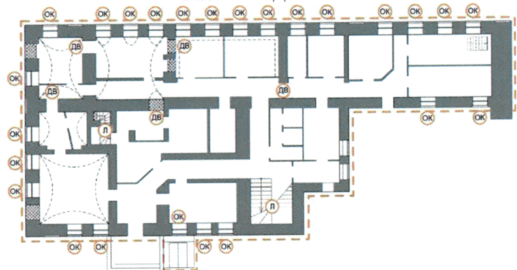
План подвала.
