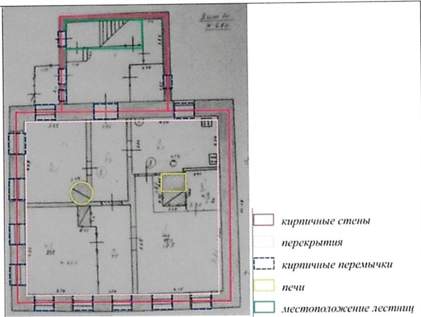
Рис. 5. Схема 1-го этажа
