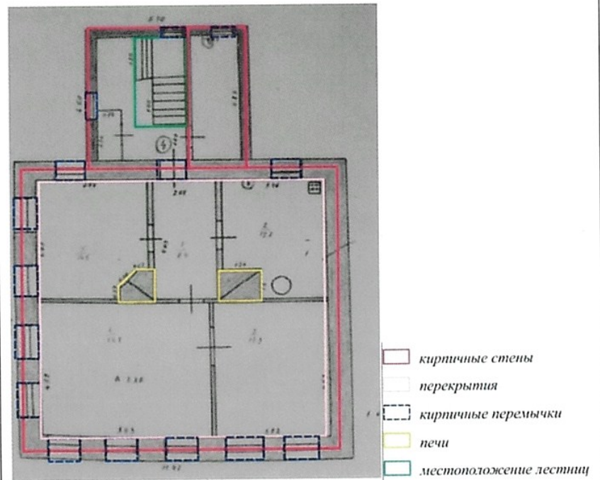
Рис. 6. Схема 2-го этажа
