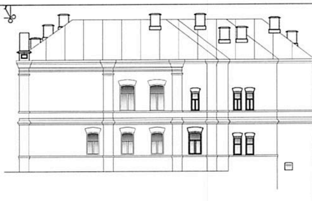
Рис 28. Восточный фасад
