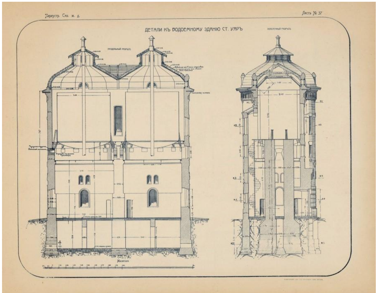
Рис. 15. Чертежи водонапорной башни на ст. Уяр. Аналог
