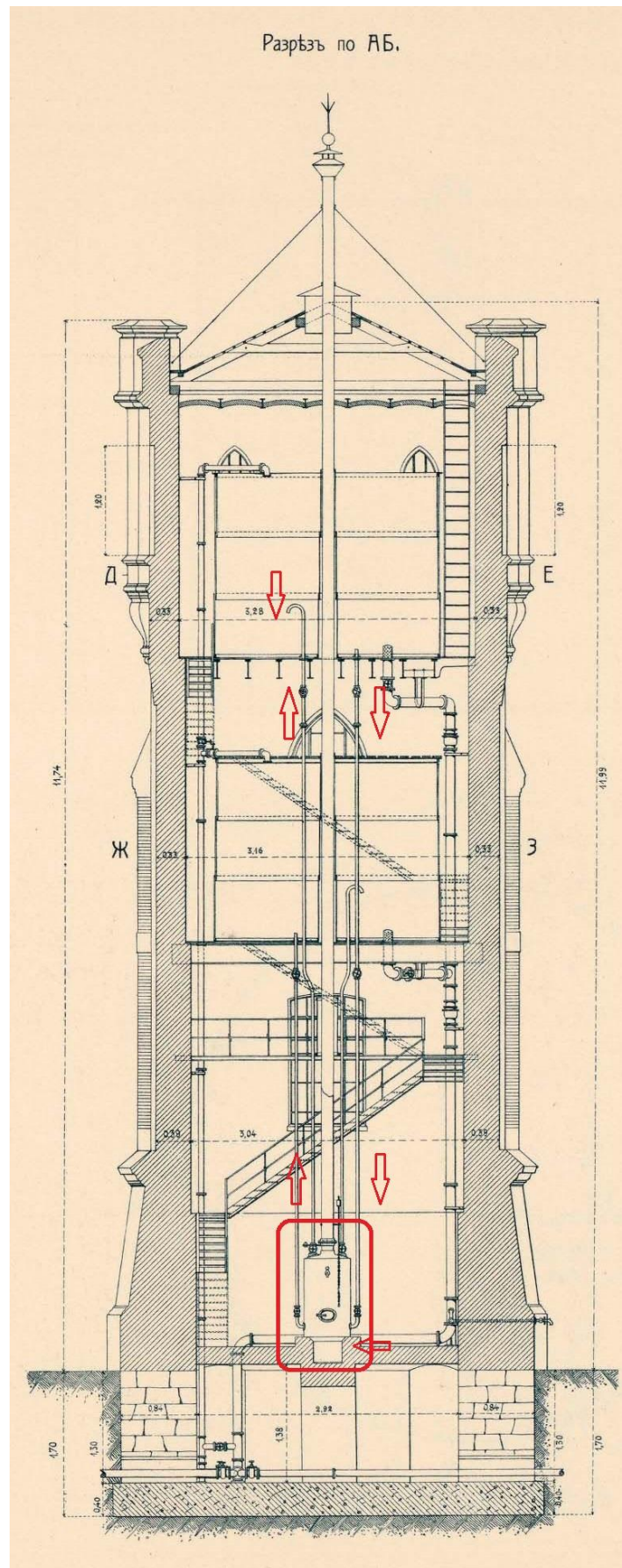
Рис. 14. Разрез водонапорной башни на ст. Лихоборы. Аналог
