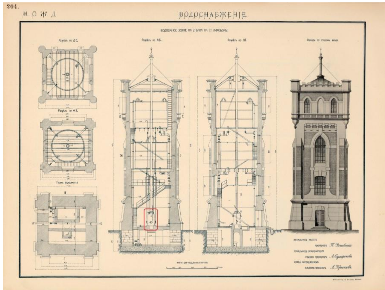
Рис. 13. Чертежи водонапорной башни на ст.Лихоборы. Аналог
