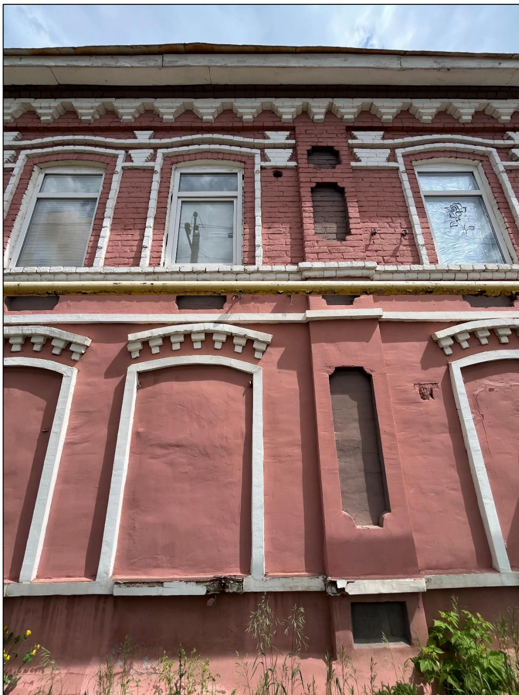
Т.ф. 4. Объект экспертизы. Ритм окон. Пилястры с фигурными нишами, венчающий карниз с городчатым поясом.
