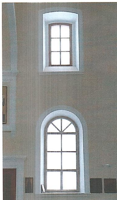
Фрагмент интерьера. Южная стена. – лучковый оконный проем 2 –ого яруса с обрамлением – 4 шт; – полуциркульные оконные проемы 1–ого яруса с обрамлением (пропорции и размеры) – 6 шт.
